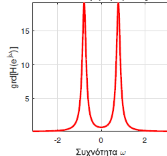
Καθυστέρηση Ομάδας
