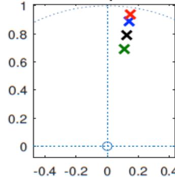
Διάγραμμα Πόλων-Μηδενικών
